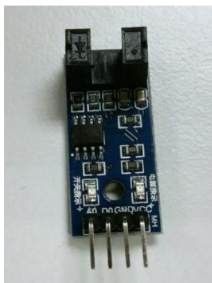
Obrázek 5: Optická závora
